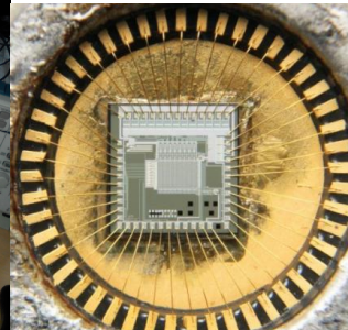
Кристал мікропроцесора під мікроскопом
