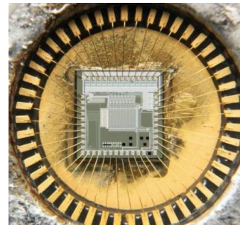
Кристал мікропроцесора під мікроскопом
